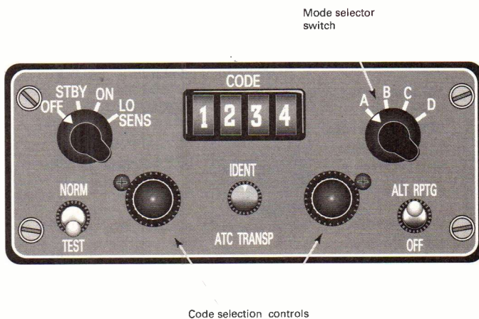
Fig. 3: Collins 621a ATC Transponder.
